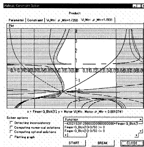
(b) 減速比 = 1/931
