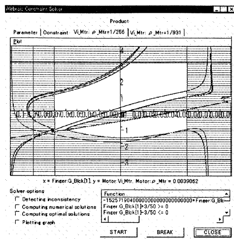
(a) 減速比 = 1/256
