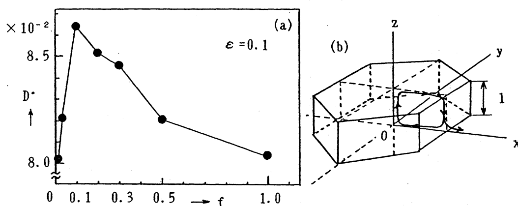
図4(a) 拡散係数の攪乱
