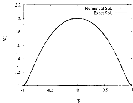
(a) N = 200 , 倍精度
