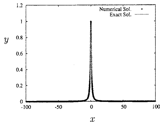
図 2. 問題 2 の解のグラフ (倍精度, \Delta x = 0.02 , 最大誤差 \sim 10^{-4} )
