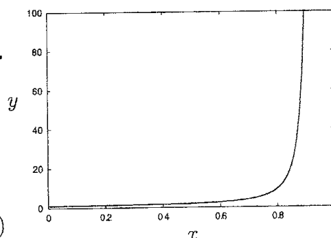
図 12. 問題 3' の厳密解のグラフ
