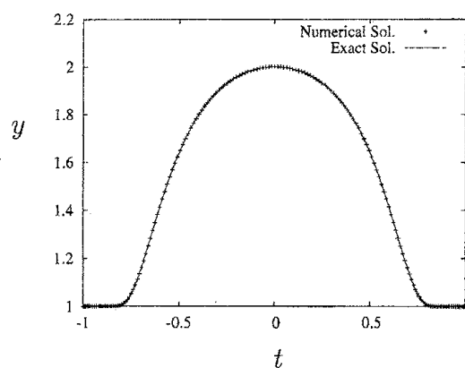
(b) N = 200 , 4 倍精度
