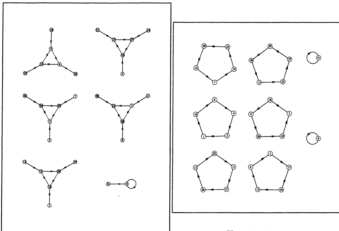
图 2: CA_{240}(5)
