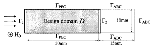
図 1 設計領域および境界条件
