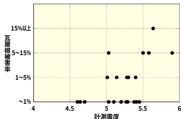
図1 観測記録の計測震度値と周辺家屋の瓦屋根被害率の関係
