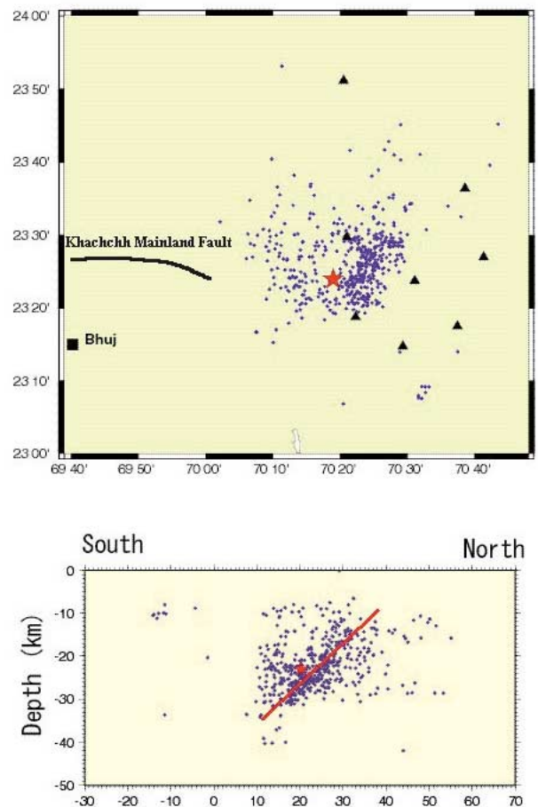
5. この研究の結果わかった余震の分布。下図の線は、南側に傾斜している断層面の方向を示している
