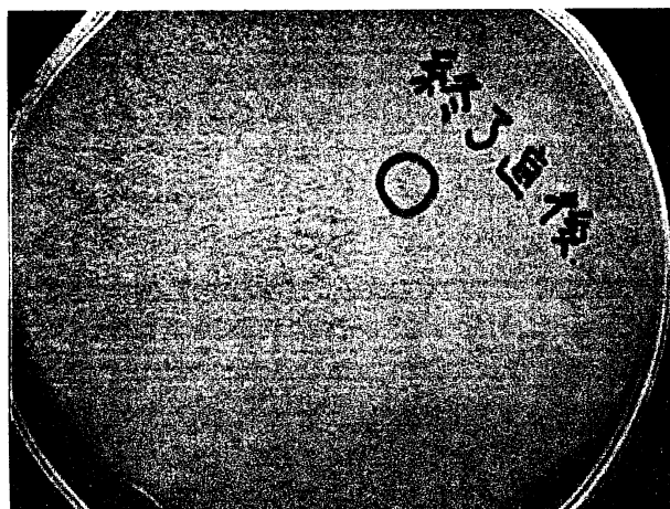
（図 14-a）時空パターン終了直後のマクロパターン。図中○印の領域を固定して顕微鏡観察。
