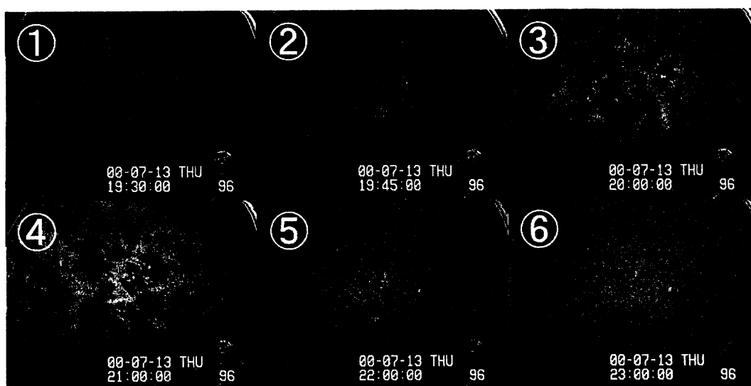
(図5)時空パターンが起こり始めてから、終わるまでの様子。①はパターンが現れはじめたところで、②、③、④の順に広がって行き、やがて⑤、⑥のように終了していく。①～④を時空パターンと呼び、③、④の時に特徴的パターンとしてストライプ、ターゲット、回転するスパイラル等が見られる。
