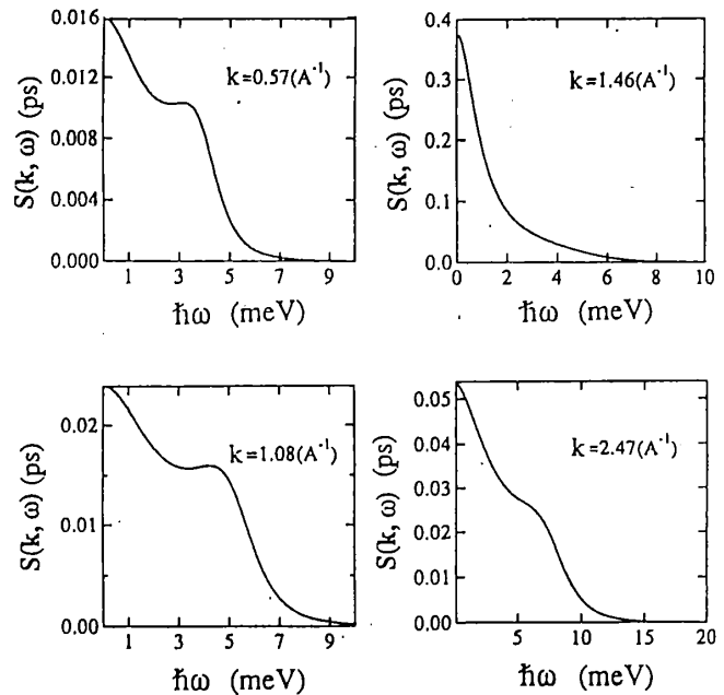
図1 液体Rbの動的構造因子 S(k, \omega) ( T=900\text{K} )
