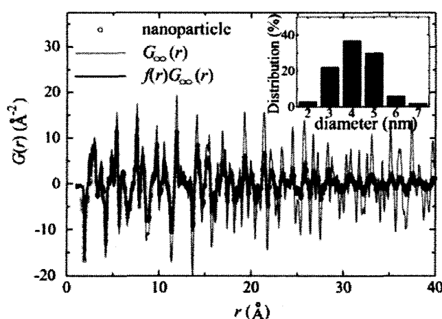
図 20. アナターゼ型 \text{TiO}_2 ナノ粒子のバルス中性子回折で得られた RPDF (○), 灰色の線はバルクの \text{TiO}_2 の RPDF と実線はそれをナノ粒子形状因子で補正した RPDF.
