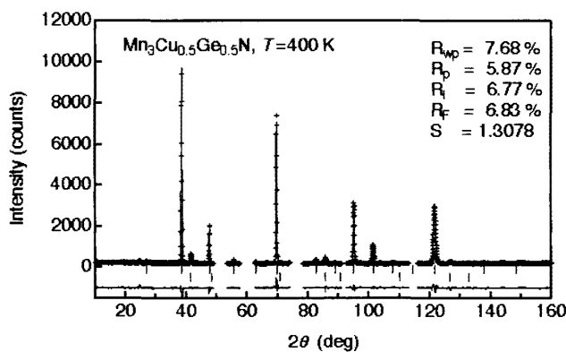
図 1 1. \text{Mn}_3\text{Cu}_{0.5}\text{Ge}_{0.5}\text{N} (400 K) の回折パターンの実験値 (×), Rietveld 解析による計算値 (実線), およびその差 (下部の細線)。
