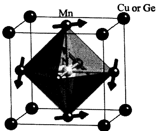
図 1 0. \text{Mn}_3\text{Cu}_{1-x}\text{Ge}_x\text{N} の結晶構造および大きな磁気体積効果を示す組成で共通して見つかった \Gamma^{5g} 型反強磁性磁気構造。Mn 6 N 八面体頂点のマンガンサイトに磁気モーメント（矢印）が存在する。
