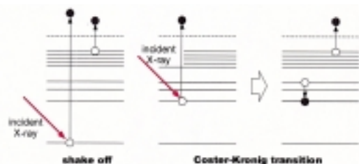
図1/二重電離状態
