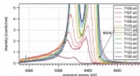
図3/FeのK吸収端近傍でのFe K \alpha_{1,2} のプロファイル差
