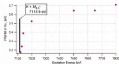
図2/K殻とM殻の電子によるshake-off過程
