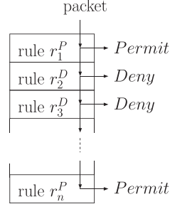
図 1: パケット分類モデル
