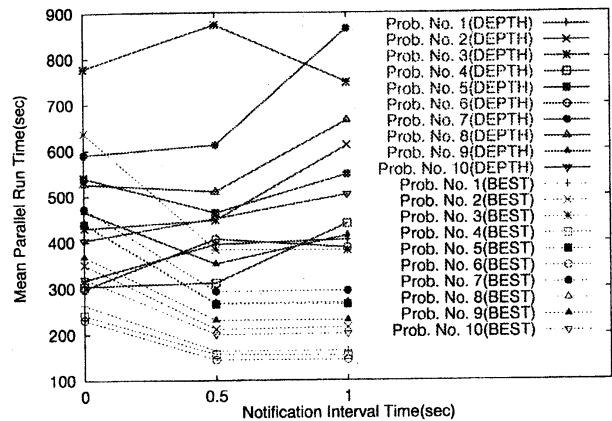
図 10: 転送方式の違いによる比較 (計算時間)
