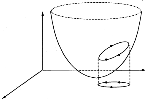
図 9: 三角形と外接円の持ち上げ
