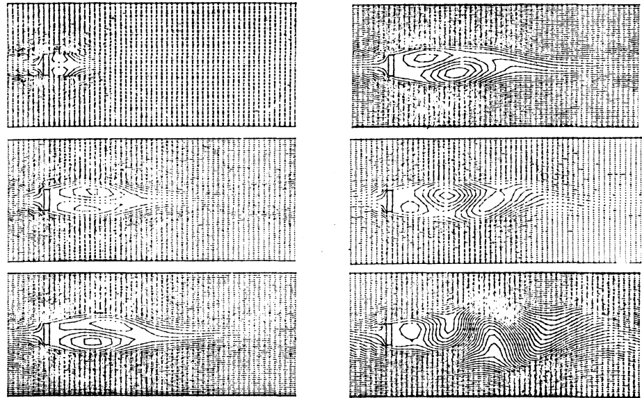
Fig. 1 : 流れの中に置かれた平板からの Karman 渦の発生 [Methods in Computational Physics, Vol. 3, p. 377 (1964) より]
