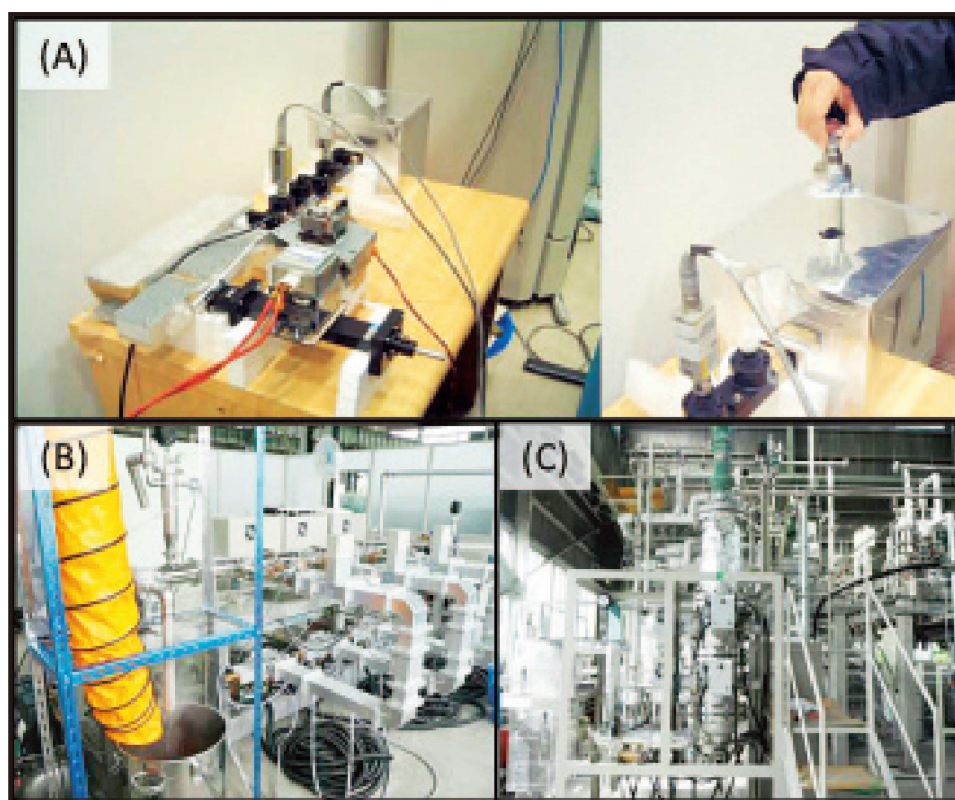
写真1 新開発のバイオマス用マイクロ波反応装置 (A): ミッション専攻研究員プロジェクト時代の反応装置 (B): 連続反応装置、(C): タワー型反応装置
