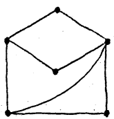
G(6,8;9)
