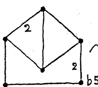
10_{104}
