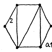
10_{45}
