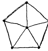
G(6,10;2) \quad 10_{123}
