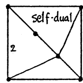
10_{115}
