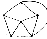
G(6,10;7) \quad (2)
