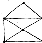
G(6,10;10) \quad (2)
