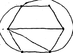
G(6,10;8)
