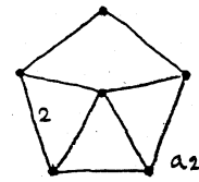
10_{117}
