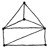
G(6,10;4) \quad (2)
