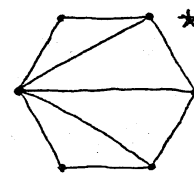
G(6,9;2)
