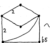
10_{81}
