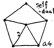
10_{118}
