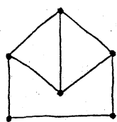
G(6,8;7)
