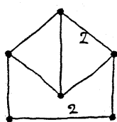
10_{84}
