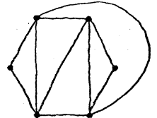
G(6,10;11) \quad (2)
