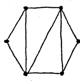
G(6,9;11)
