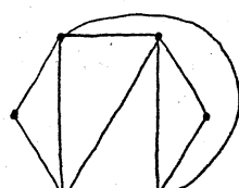
G(6,10;11)
