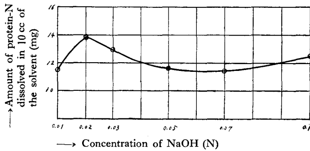
第八圖 搗磨肉 10 g に對し苛性曹達液 200 cc を用ひた場合
