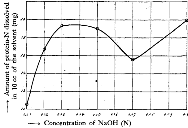
第八圖 搗磨肉 10 g に對し苛性曹達液 200 cc を用ひた場合
