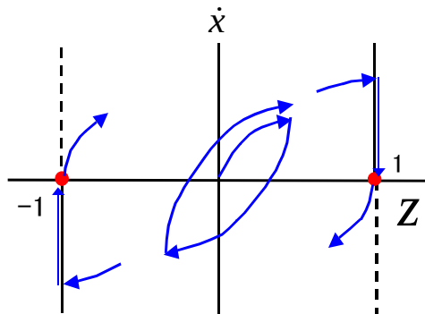
Fig. 2 Trajectory in \dot{x} - z plane
