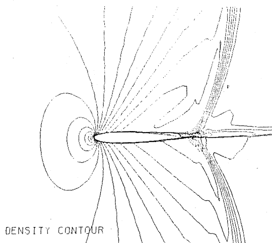
Fig.15 M=.95 , Re=10^5 .
