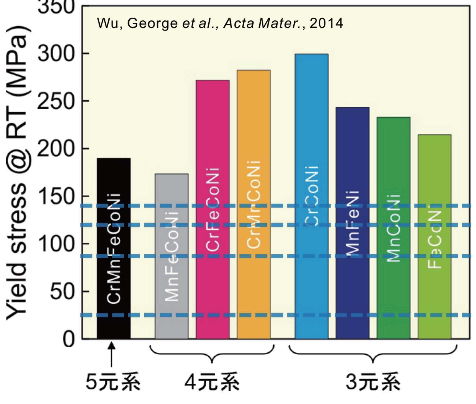
ハイレントロピーFCC合金の降伏強度
