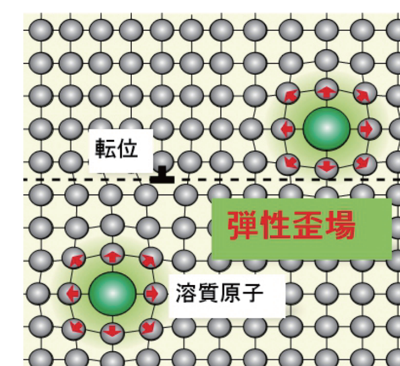
Fleisherモデル
