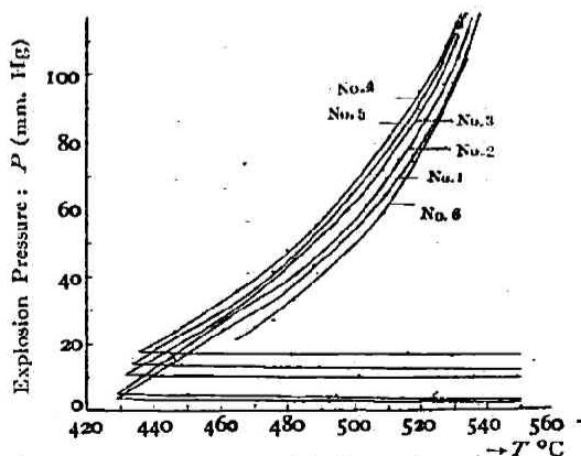
Fig. 1. Reaction tube No. 1, d=4.02 cm.; No. 2, d=3.15 cm.; No. 3, d=2.65 cm.; No. 4, d=2.07 cm.; No. 5, d=1.73 cm.; No. 6, d=1.30 cm.
