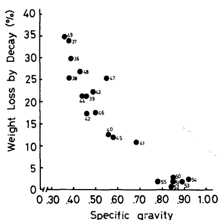
Fig. 14. Relationship between weight loss of Shorea spp. due to decay by Coriars versicolor and their specific gravity (36; Shorea fallax , 37; S. gysbertsiana , 38; S. leprosulla , 39; S. macroptera , 40; S. ovalis , 41; S. parvifolia , 42; S. platycarpa , 43; S. sp. , 44; S. sp. , 45; S. agami , 46; S. symingtonii , 47; S. sp. , 48; S. gibbosa , 49; S. hopeifolia , 50; S. exelliptica , 51; S. hypoleuca , 52; S. laevis , 53; S. leptoderma , 54; S. sp. , 55; S. sp. ) (36~44; red meranti, 45~47; white meranti, 48~49; yellow meranti, 50~55; Selangan batu).
