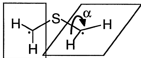
図2. (Ia) のコンフォメーション変化
