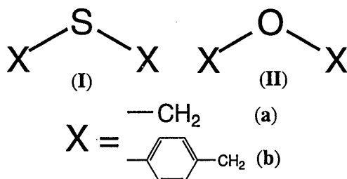
図1. (Ia), (Ib), (IIa), (IIb) の図
