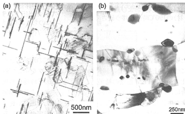
図1 時効熱処理を行ったAl-2 mass%Cu合金のTEM組織。(a)通常粒径材(溶体化材)。溶体化、水冷後、190℃で108 ks時効。(b)超微細粒材。溶体化、水冷後、室温で6サイクル(相当圧下ひずみ4.8)のARBを行ったのち、190℃で108 ks時効。
