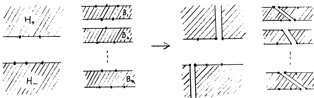
図 6. R_0 の分割
