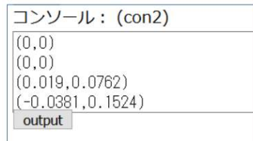
図 8 : 実行画面
