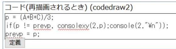
図 7 : CindyScript の命令
