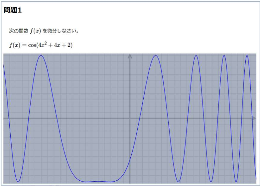
図 5 : 実行画面
