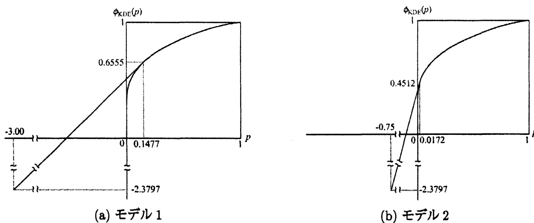
図 3: 核型密度推定に基づいた最適ソフトウェア若化スケジュールの推定
