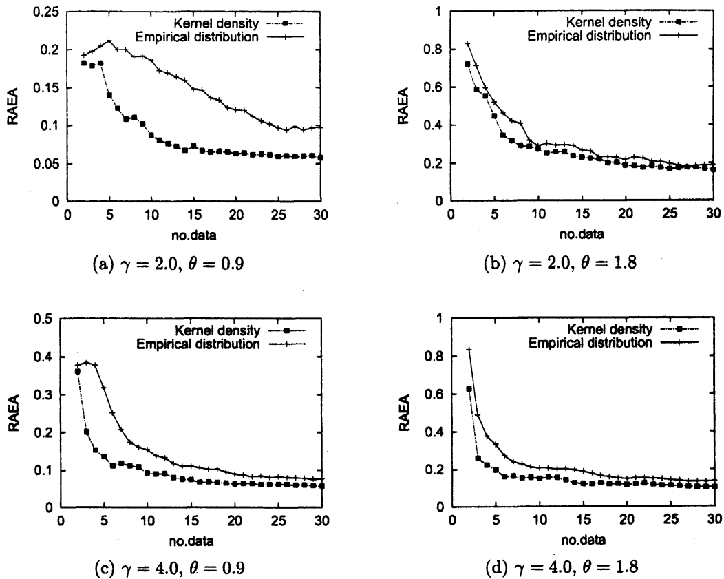
図 7: 最適ソフトウェア若化スケジュールの推定値に関する相対絶対誤差平均 (モデル 2)
