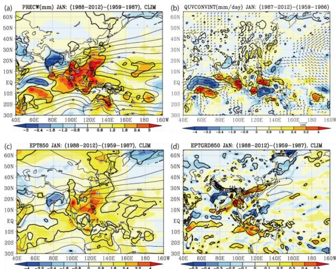
図 3. 1 月の後期－前期(色)と気候値(実線). (a)可降水量(mm), (b)鉛直積算水蒸気フラックスの後期－前期(矢印, mm m/s)と収束(mm/day). (c)850hPa の相当温位(K)と(d)水平勾配(K/100km).
