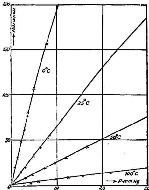
第 三 圖 吸着恒温曲線 ( \text{CO}_2 , 精製炭)
