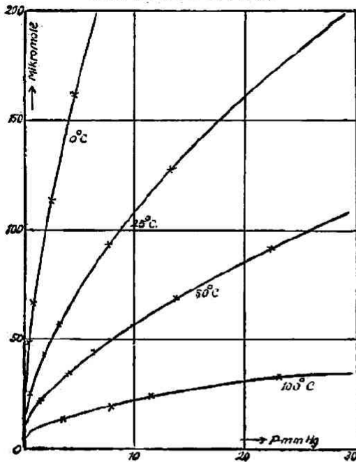
第 四 圖 吸着恒温曲線 ( \text{CO}_2 , 不純炭)
