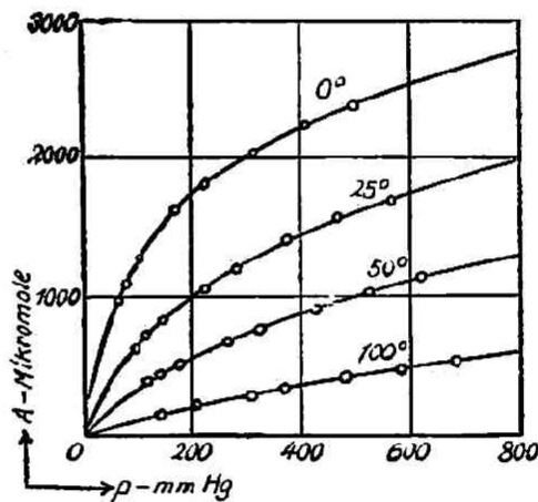
第 一 圖 \text{CO}_2 恒温曲線（高壓）
