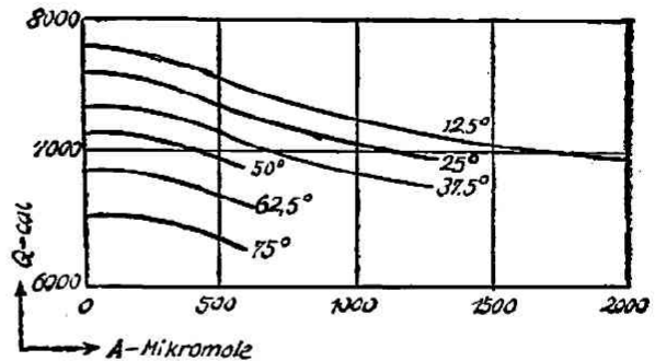
第 二 圖 吸着熱 ( \text{CO}_2 , 精製炭)
