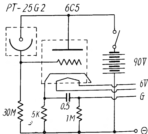
光電管ユニット配電図
