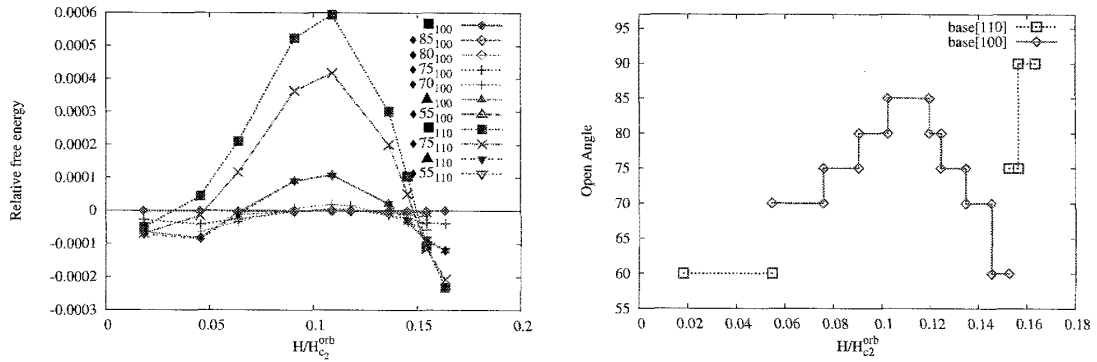
図8 \bar{\mu} = 2 , 温度 T/T_c = 0.2 における (左) 相対エネルギーの磁場依存性と (右) 開口角の変化.
