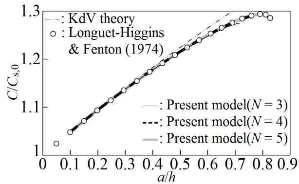
図-2 相対位相速度 C/C_{s,0} ( C_{s,0} は、線形浅水波の位相速度である。)
