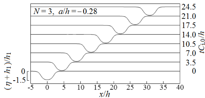
図-6 進行する内部孤立波の界面形の時間変化 ( \rho_2/\rho_1=1.02; h_1/h=0.2 )
