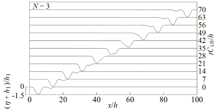
図-7 振幅の異なる二つの内部孤立波の追い越し ( \rho_2/\rho_1=1.02 ; h_1/h=0.2 |a|/h_1=1.4 and 0.3 )
