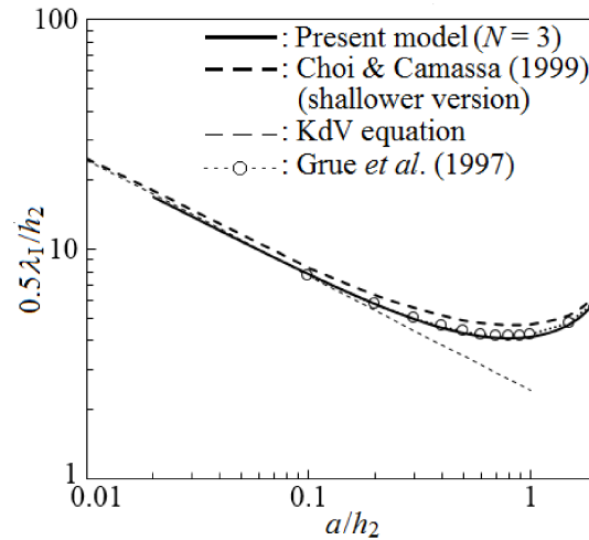
図-4 相対代表半波長 0.5\lambda_1/h_2 (密度比 \rho_1/\rho_2=0.63 , 静水時の上層厚 h_1=0.836h )
