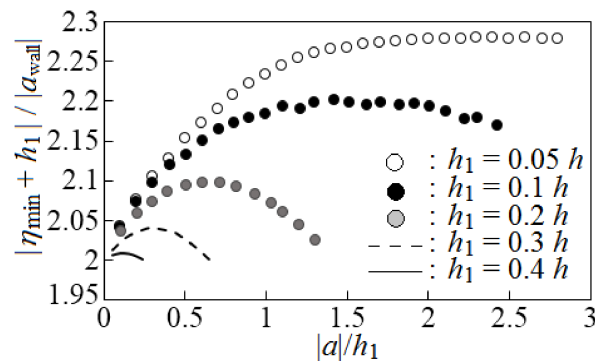
図-8 内部孤立波が鉛直壁に衝突する場合の波高上層厚比 |a|/h_1 と波高増幅率 |\eta_{\min} + h_1|/|a_{\text{wall}}| の関係 ( N=3 )
