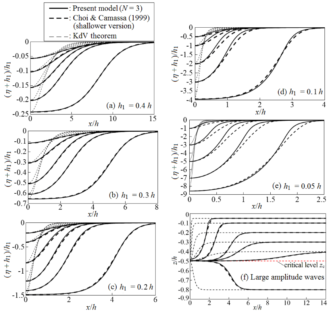
図-3 内部孤立波の界面形の数値解と理論解
