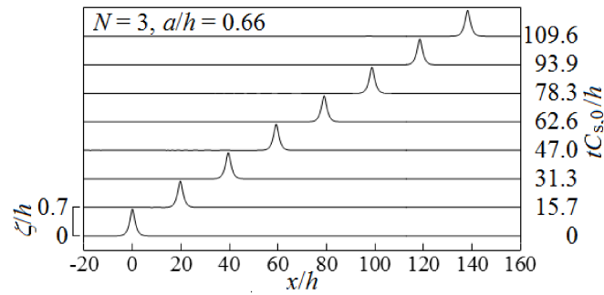
図-5 進行する表面孤立波の水面形の時間変化
