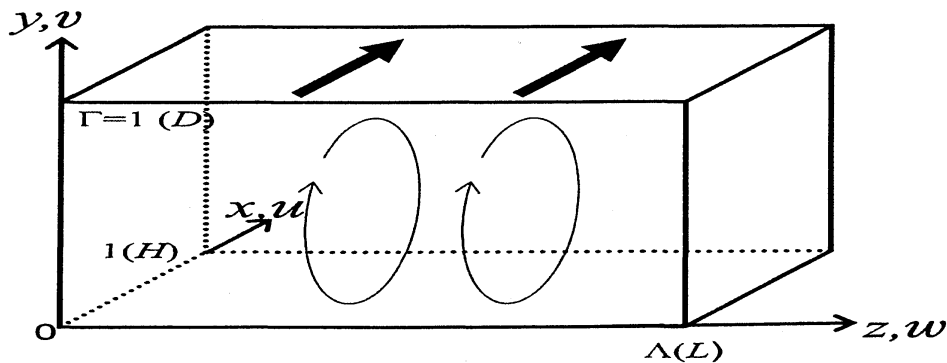
図 1 座標系と面の運動の概略図
