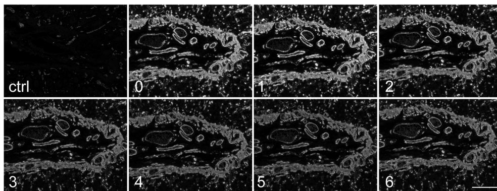
b MUGF3
