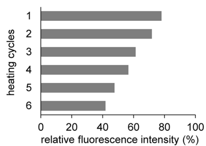
MUGF3
