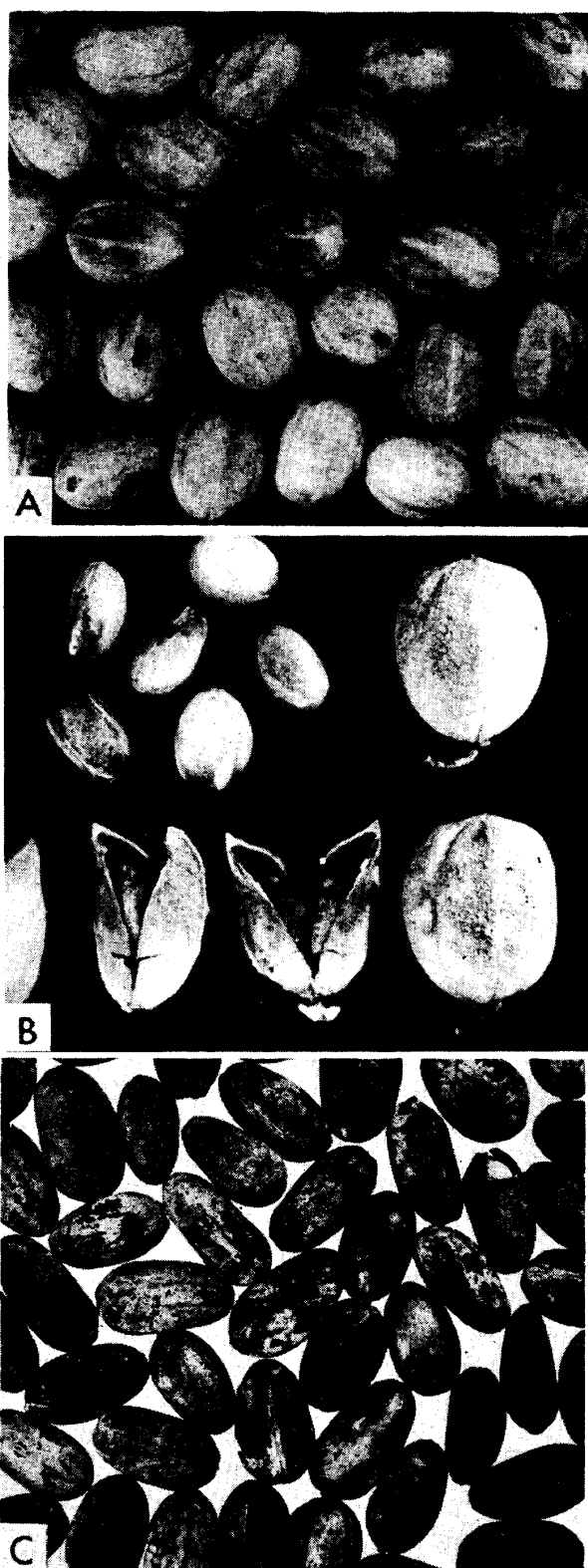
写真 Sd-22 “Sa lod” (巴豆) A：果実（果皮をともなった種子） （巴豆）（ca. \times 0.7 ） B：裂開した果実（ca. \times 1.2 ） C：種子（巴豆，巴米）（ca. \times 1.1 ）
