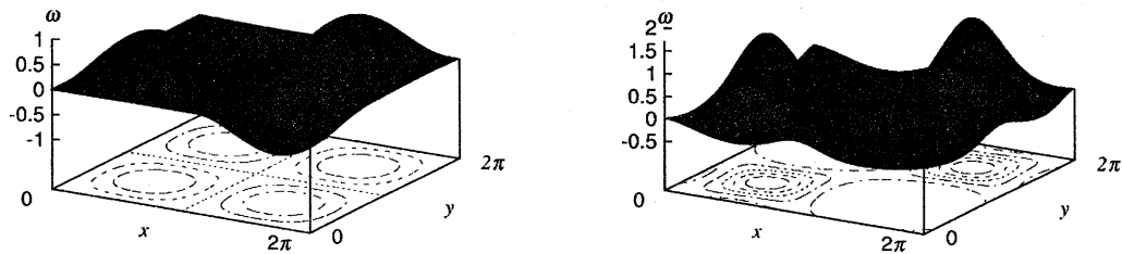
Fig.3(a): t=0 における \omega の鳥瞰図および等高線 (b): t=0.6 . 高線.
