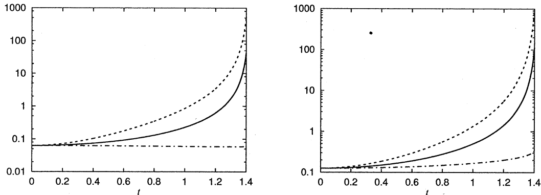
Fig.1(a): ノルムの時間発展 E_\omega(t) (一点鎖線), E_\gamma(t) (実線) および E_W(t) (破線). Fig.1(b): Q_\omega(t) (一点鎖線), Q_\gamma(t) (実線) and Q_W(t) (破線) の時間発展.
