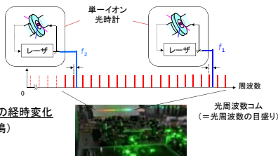
2種類の単一イオン光時計の周波数比較
