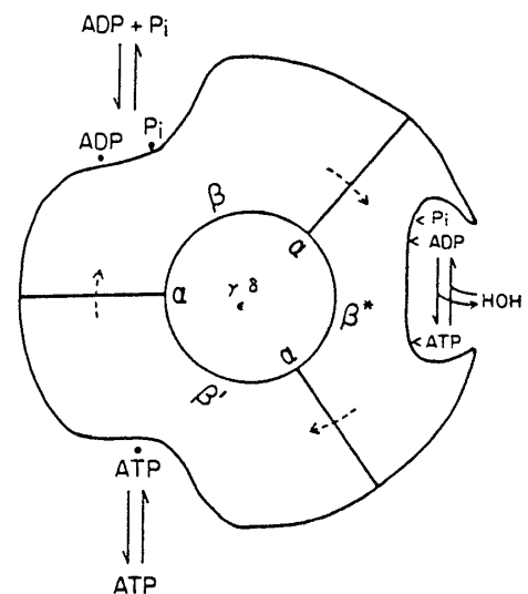
図3. Boyer らの alternating three-site モデルの模式図。
