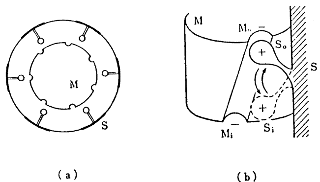
図5. (a)回転モデルにおける F_0 の予想される構造。十数個のサブユニットcが外筒Sを作る。Sはプロトン吸脱着できるいくつかの手を持つ。2個のサブユニットbは内筒Mを作る。内筒の外面では、斜めに走る溝があり、Sの手がはまりこむことができる。(b)回転モデルにおけるルース・カップリング機構。Sから出る手は2つの位置 S_0 と S_i の間を \Delta\mu_{H^+} の駆動力に応じて往復運動する。手Sは溝Mに沿って動くことができるが、溝にはまらない確率もあるとする。(大沢(1985), 文献9より転載)。
