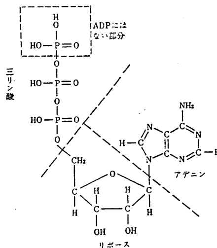
図1 アデノシン三リン酸 (ATP) の分子構造
