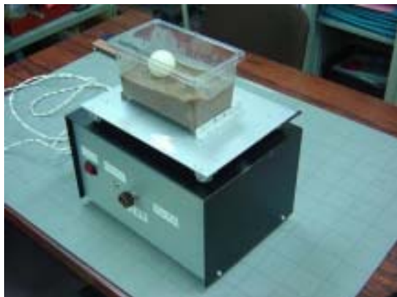
写真 2 液状化模型
