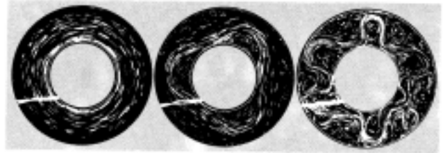
図 2. 偏西風擾乱
