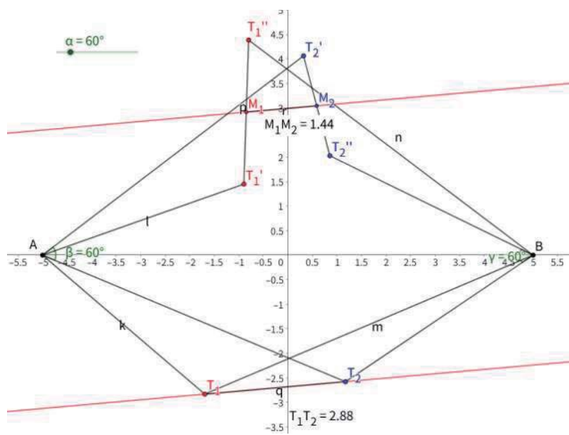
図 2 A(4) に基づく GeoGebra で作図した結果
