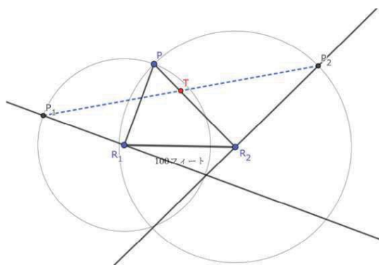
図1 点 P :ヤシの木, R_1, R_2 :岩, P_1, P_2 :海賊が立つ位置, T :宝.
