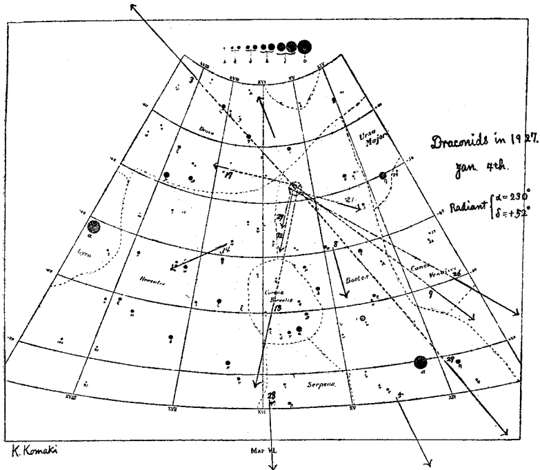
第二圖 龍座流星群の輻射點
