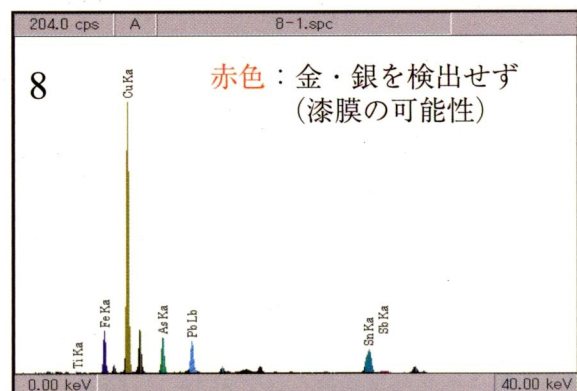
図5 XRF スペクトル (測定箇所 1, 4, 8, 14)
