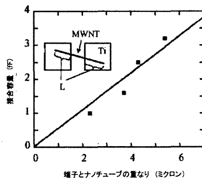
図 6 クーロンブロッケイド現象を解析して求めた接合容量と Ti 電極下ナノチューブの長さとの関係。
