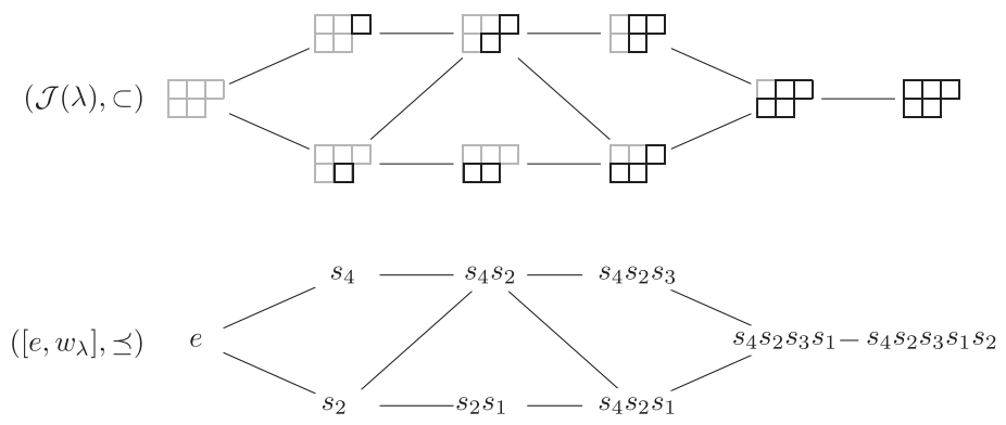
図 5 \lambda = (3, 2) に対する \mathcal{J}(\lambda) と [e, w_\lambda] の Hasse 図.
