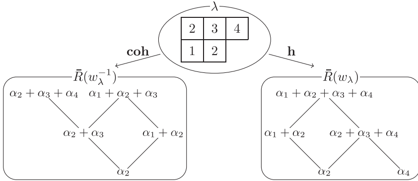
図2 \lambda = (3, 2) の Young 図における半順序構造
