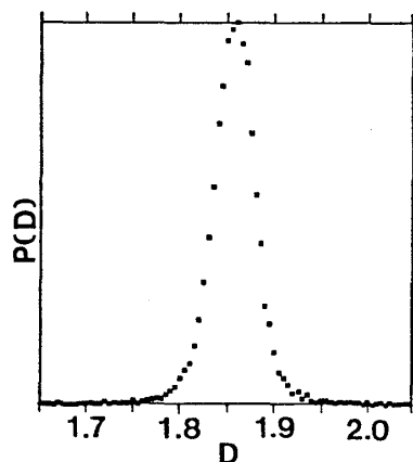
図1 2次元 Ising Model の(無限系での)臨界点での磁化でのフラクタル次元 D の分布 P(D) 。64 × 64 の系での 50 万モンテカルロステップの結果より。
