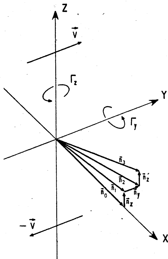
第 17 図 shear flow instability の起る概念図 （静的：DC の場合）
