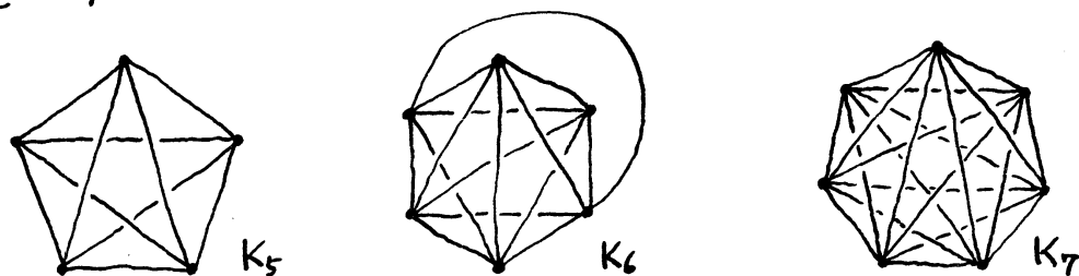
図1: 完全グラフ K_5, K_6, K_7 の射影図の一例
