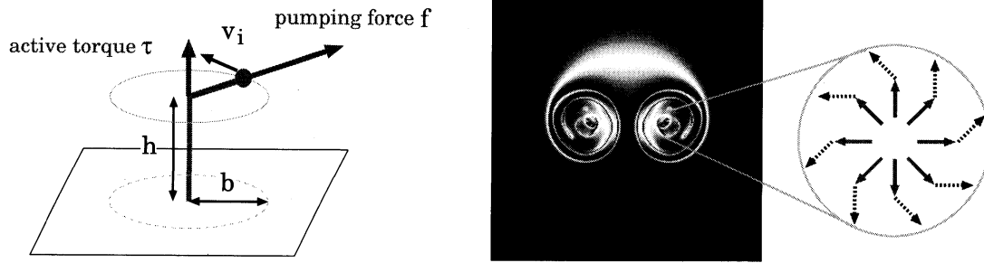
図1: (左) 回転子モデル. (右) 回転数 \pm 1 の位相欠陥の対から生じたらせん波 ( \delta = 60^\circ ). 回転子の腕が放射状になっている場合, 反時計回りのらせん波が生じる.
