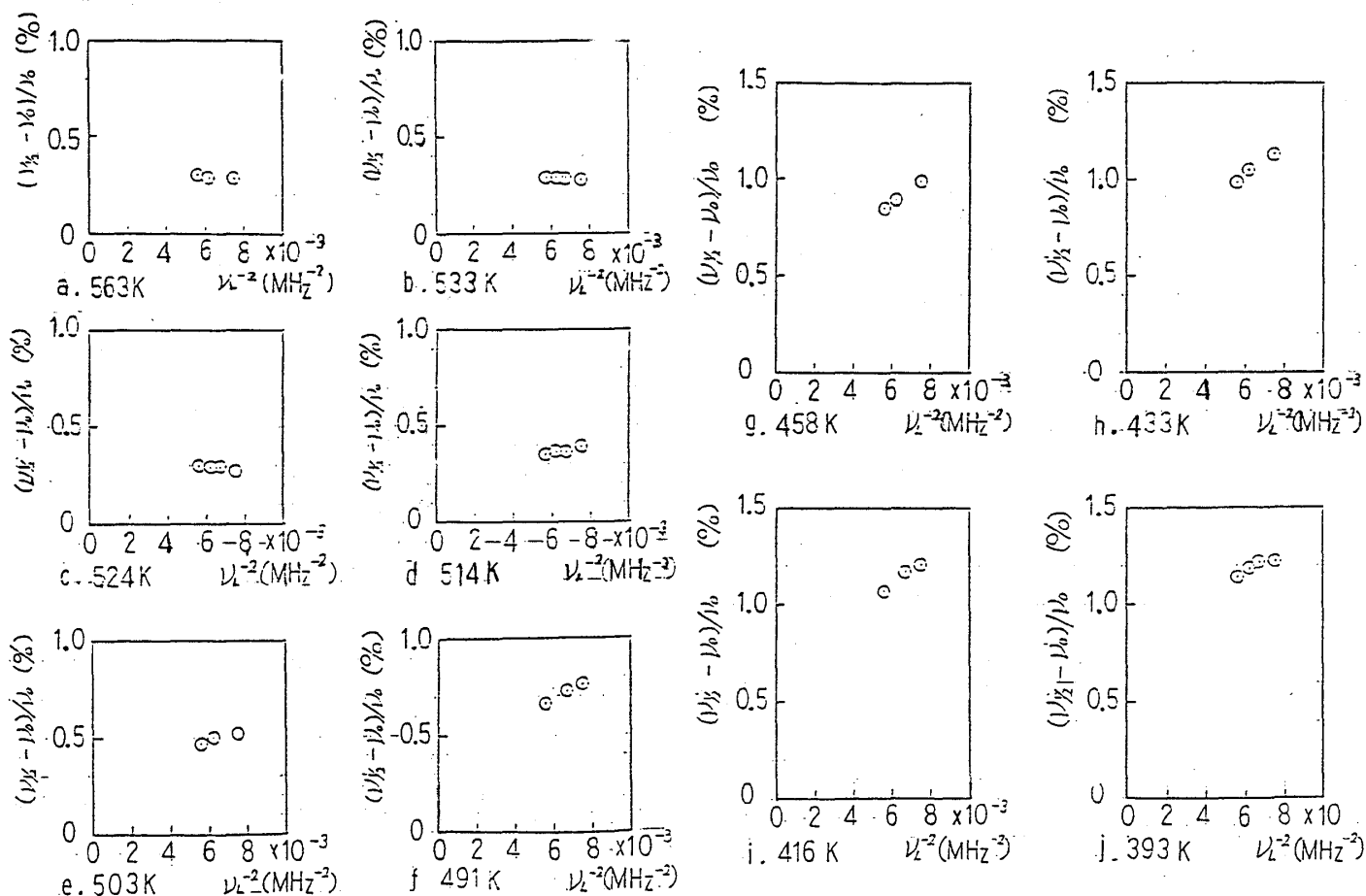
図3-17 Bi核のシフトと周波数の関係 ( C \parallel Ho )
