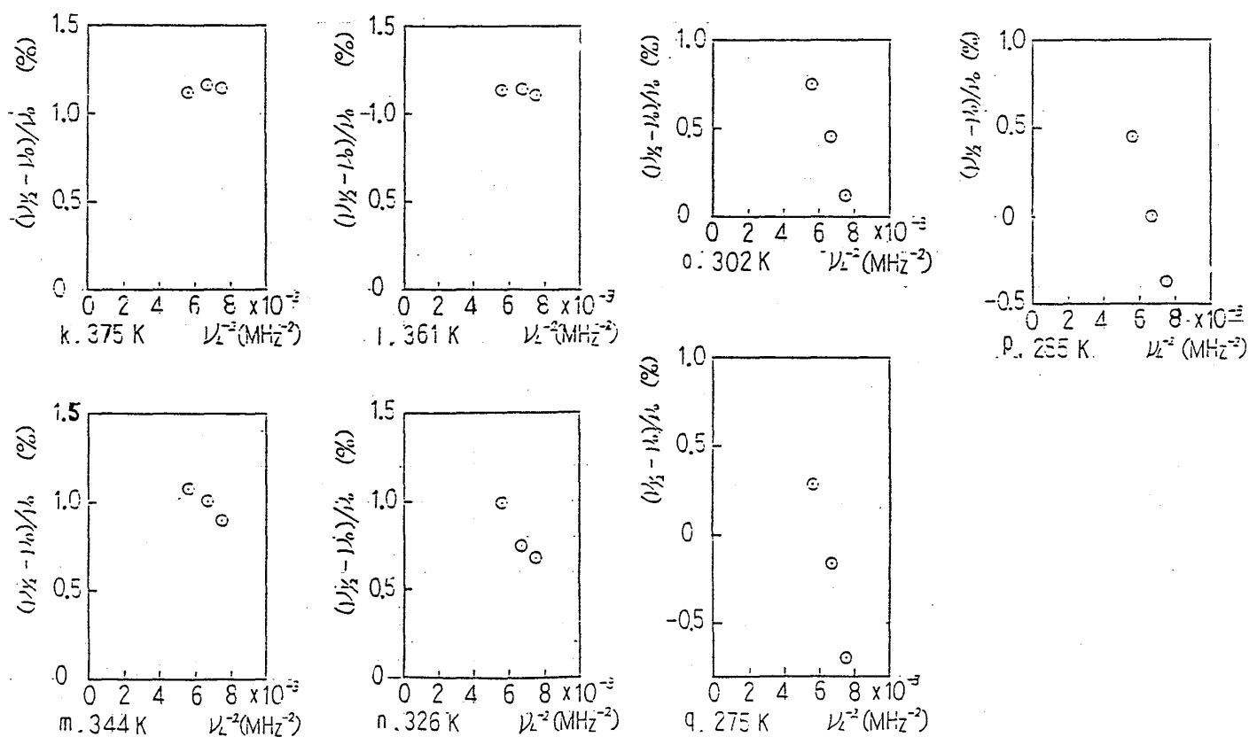
図3-18 Bi核のシフトと周波数の関係 ( C \parallel Ho )
