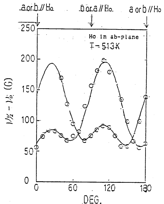
図 3-22 \text{Bi} 核の中心線の角度変化
