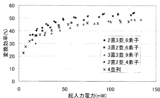
図2 各接続数における140Ω抵抗接続時の変換効率
