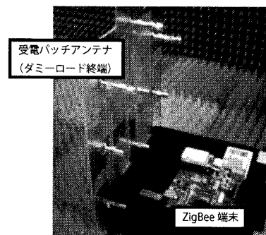
図3 受電アンテナによる遮蔽
